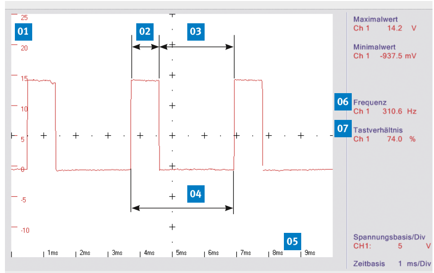
Exemple : signal PWM avec un rapport cyclique de 74%
